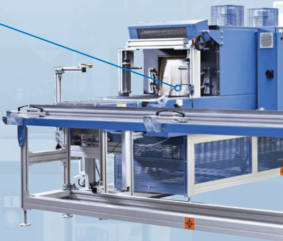
Bezúdržbový tunelový dopravník s akumulčním koncovým dopravníkem s počítačací funkcí
