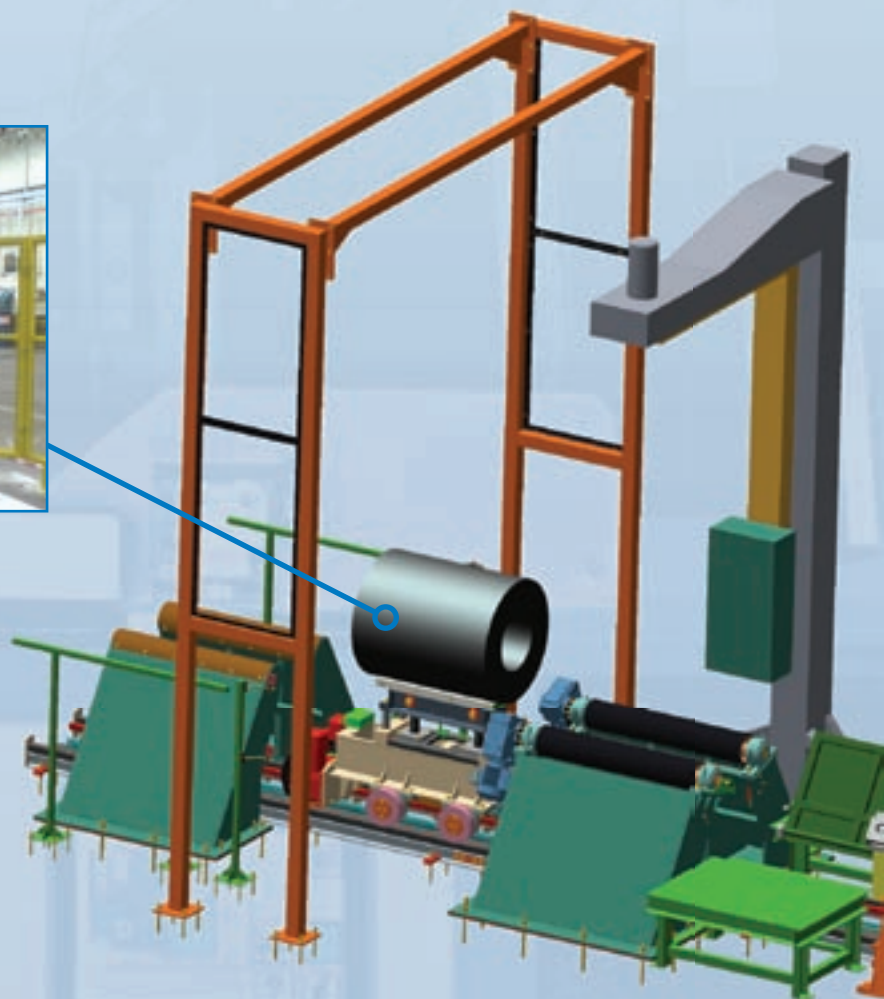
Balicí linka svitků pocínovaných plechů se zakládacím hydraulickým vozíkem, ovinovacím automatem a s překlápěčkou zabalených svitků
