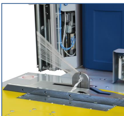
Automatické uchycení řezání a zažehlení fólie
